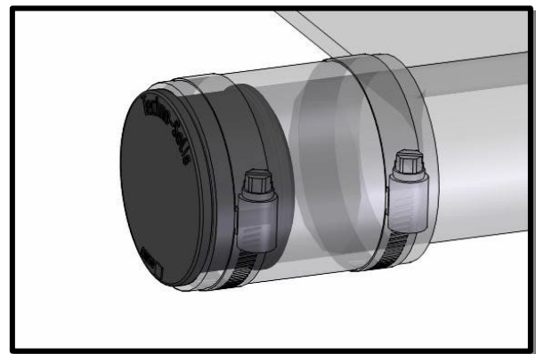
9. Tapón de Extremos
