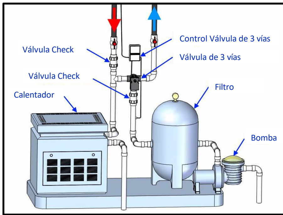
14. Instalación en el cuarto de máquinas del sistema
